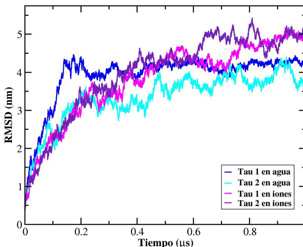
FIGURA 7. RMSD para ambos sistemas tau. El sistema taus-agua corresponde a las líneas azul y cian. El sistema taus-iones se muestra con las líneas magenta y lila.
