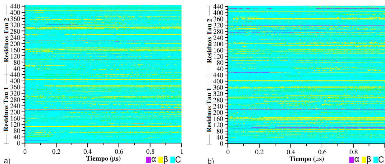
FIGURA 5. Estructura secundaria correspondiente a los dos monómeros tau con 441 aminoácidos para los sistemas a) taus-agua y b) taus-iones. El color lila muestra las hélices- \alpha ; el amarillo las hojas- \beta y el cian las espirales aleatorias.
