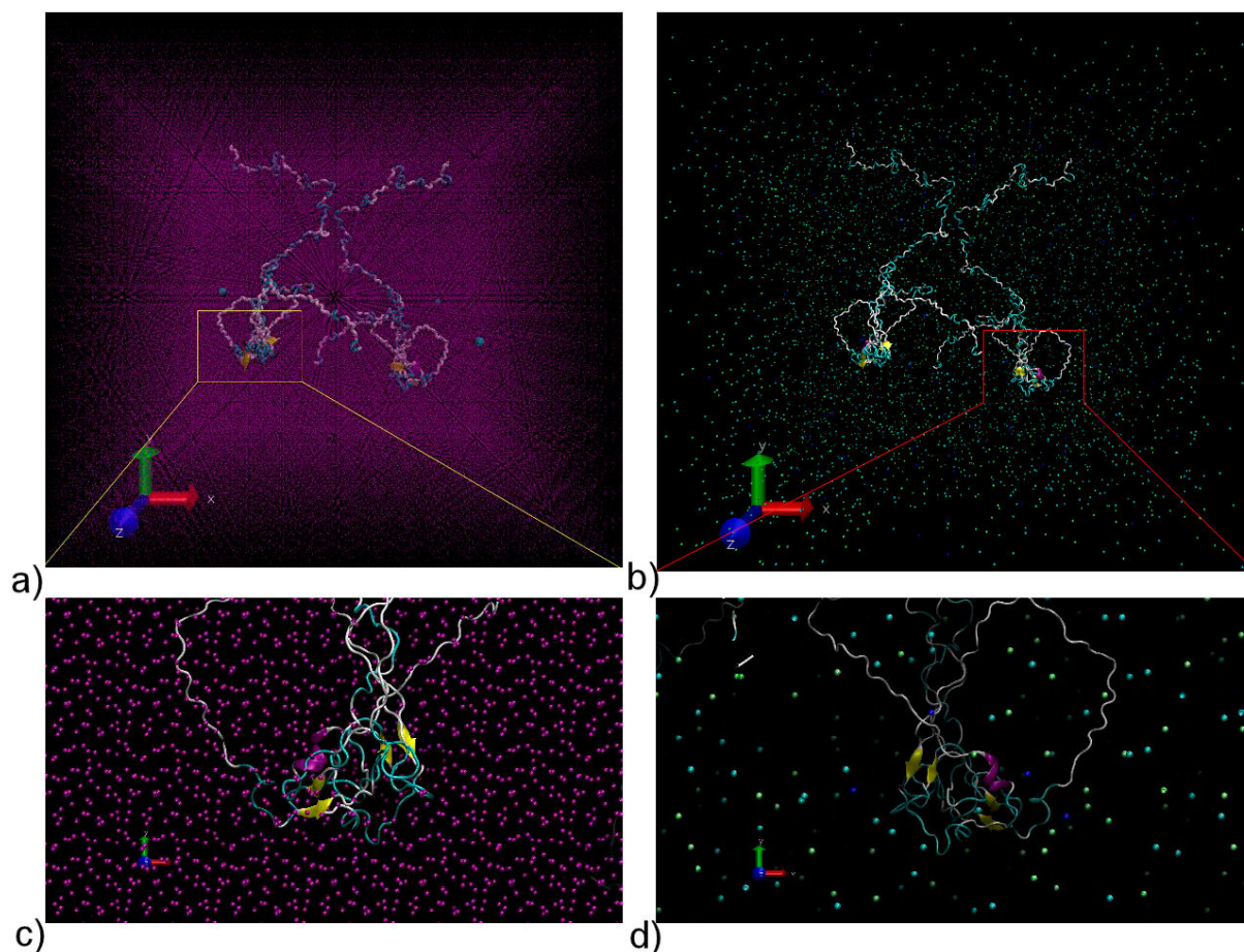
FIGURA 2. Representación visual atómica de los dos sistemas tau: a) dos monómeros tau con solvente explícito y b) dos monómeros tau en solvente explícito y en presencia de iones. En este sistema se omitió el solvente para una visualización más clara de los iones. c) Sección ampliada de las tau en únicamente agua y d) sección ampliada de las tau en iones. En ambos sistemas se observan hélices- \alpha y láminas- \beta . La representación de estas estructuras se realizó con VMD y la herramienta sirah.backmap de SIRAH Tools [43,44].
