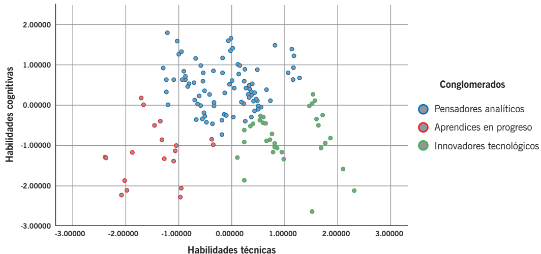
Figura 4. Dispersión agrupada de habilidades cognitivas y técnicas Fuente: elaboración propia en SPSS a partir de los datos.
