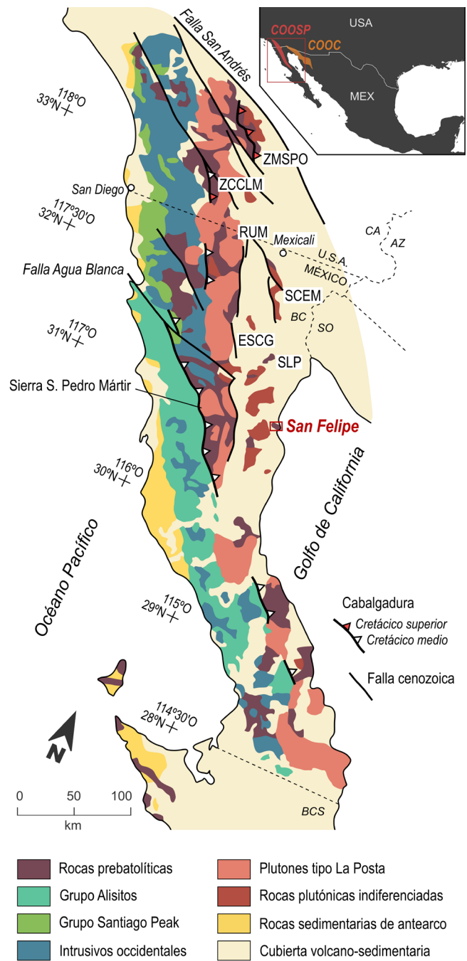
Figura 1 Mapa geológico simplificado del batolito de las Sierras Peninsulares modificado a partir de Kimbrough et al. (2001). En el cuadro de la esquina superior derecha se muestra la localización de los cinturones de oro orogénico del noroeste de México. Abreviaturas: ESCG, Escarpe del Golfo; RUM, La Rumorosa; SCEM, sierras Cucupá-El Mayor; SLP, sierra Las Pintas; ZCCLM, zona de cizalla Cuyamaca-Laguna Mountains; ZMSPO, zona milonítica de las Sierras Peninsulares Orientales; (estados) AZ, Arizona; BC, Baja California; BCS, Baja California Sur; CA, California; SO, Sonora.
