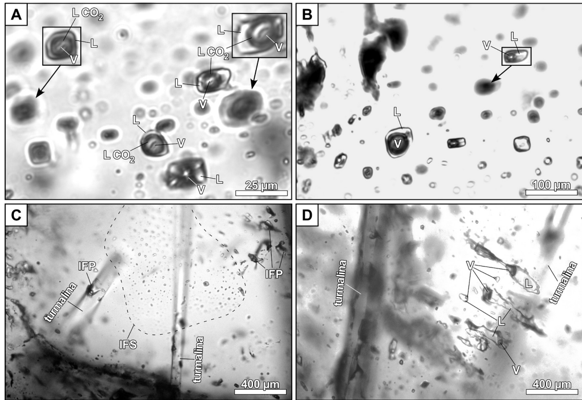
Figura 6 Fotomicrografías de asociaciones de inclusiones fluidas (AIF) representativas en cuarzo del depósito sinorogénico de oro de La Felipeña. (A) AIF primaria consistente en inclusiones bifásicas ricas en líquido (L+V) e inclusiones con fluidos inmiscibles (salmuera acuosa y CO 2 ) indicativa de atrapamiento heterogéneo, vg. medio en que la precipitación mineral se puede vincular a efervescencia. (B) AIF primaria con morfologías tendentes a cristal negativo y grado de relleno homogéneo. (C y D) AIF primarias en asociación con cristales de turmalina, que presentan inclusiones de grandes dimensiones con grado de relleno homogéneo; muchas de las inclusiones primarias se encuentran en los bordes de grano entre cuarzo y turmalina. Clave: IFP = inclusiones fluidas primarias, IFS = inclusiones fluidas secundarias, L = líquido, V = vapor.
