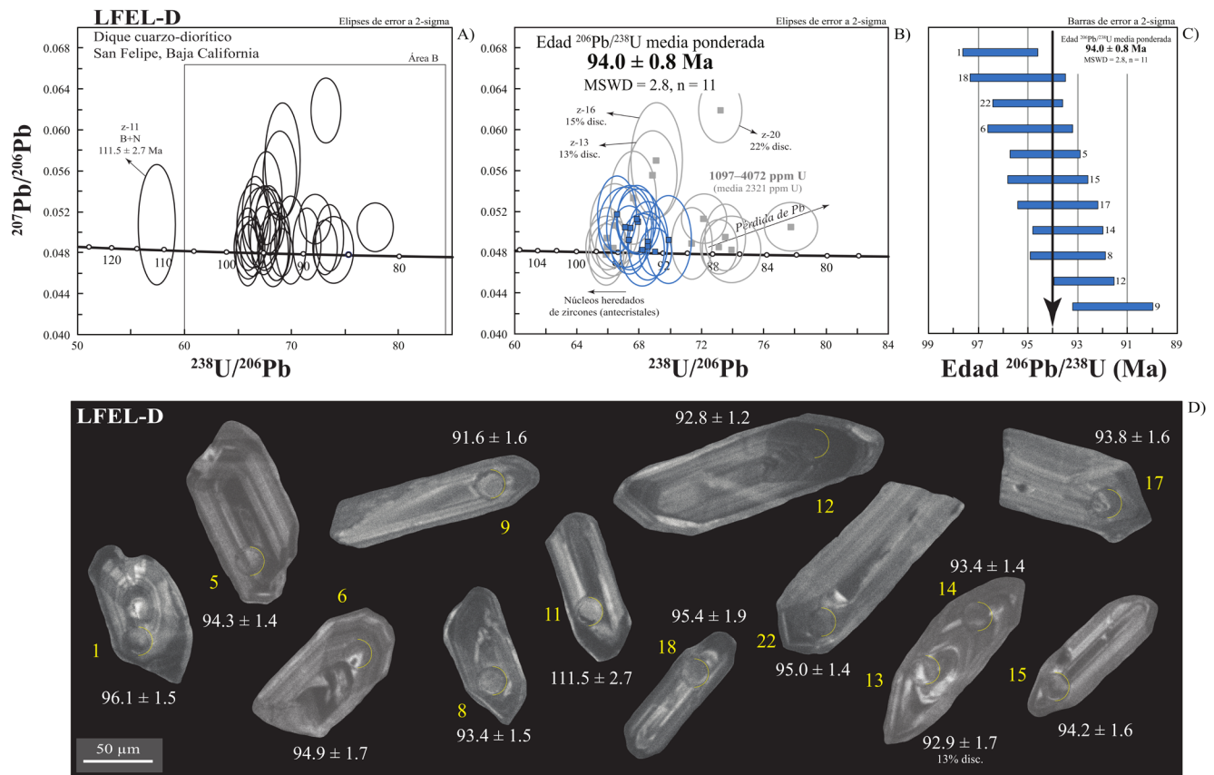
Figura 4 Gráficos de datos U-Pb obtenidos mediante la técnica de ablación láser (LA-ICP-MS) e imágenes de catodoluminiscencia de los circones del dique cuarzo-diorítico del prospecto La Felipeña. El procesamiento de los datos se realizó con el esquema de reducción de datos “VizualAge” (Petrus y Kamber, 2012) para el software “Iolite 2.5” (Paton et al. , 2011). (A) Diagrama de concordia tipo Tera-Wasserburg mostrando todos los datos de los circones analizados de la muestra LFEL-D. (B) Acercamiento a los datos más jóvenes en donde se muestra la edad ^{206}\text{Pb}/^{238}\text{U} media ponderada calculada. (C) Diagrama de media ponderada mostrando los análisis utilizados para calcular la edad media ponderada. Las elipses de color azul representan los análisis utilizados para el cálculo de la edad media ponderada, mientras que las elipses de color gris representan los datos que fueron descartados para el cálculo de la edad media ponderada debido a que corresponden a circones con un cierto grado de pérdida de Pb, herencias (antecristales) o, simplemente, altos grados de discordancia. (D) Imágenes de catodoluminiscencia post ablación láser de algunos circones representativos utilizados para el cálculo de la edad media ponderada, donde los medios círculos amarillos corresponden al lugar de ablación de un diámetro de \sim 22 \mu\text{m} .
