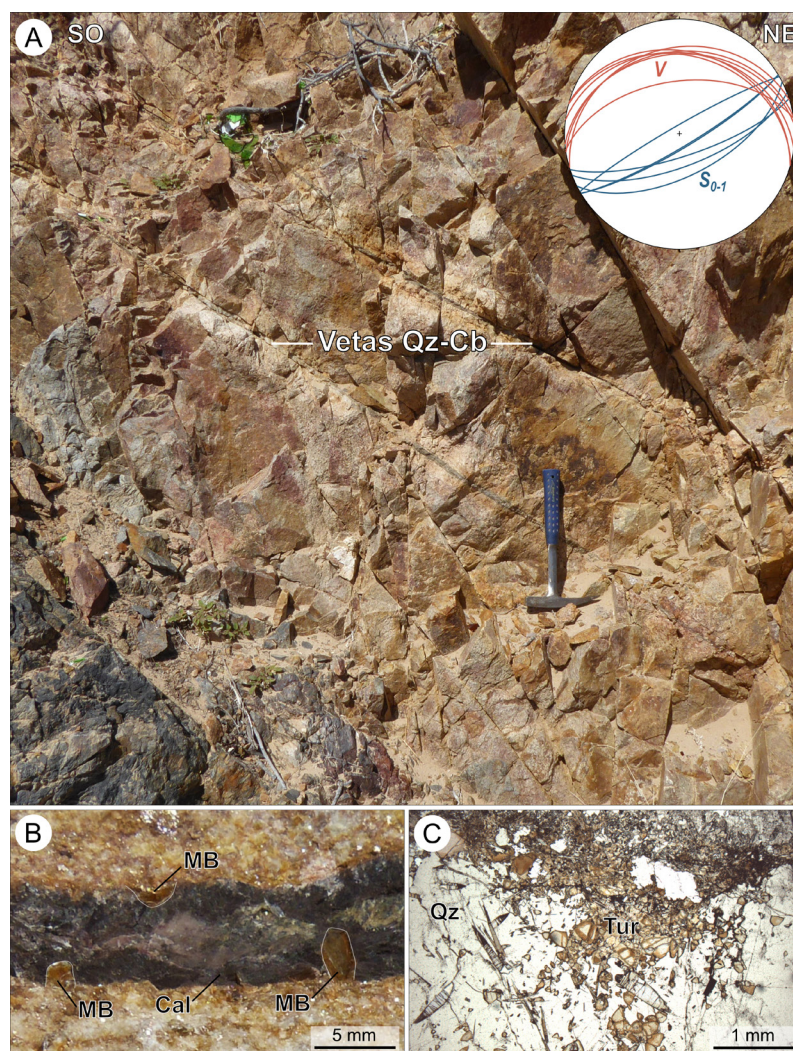
Figura 3 Rasgos representativos de la mineralización del prospecto La Felipeña. (A) Vetvas extensionales subparalelas de cuarzo-carbonato alojadas en la zona de contacto entre un dique cuarzo diorítico (subconcordante) y metaargilitas (esquina inferior izquierda). Las muestras para los análisis geocronológicos (LFEL-V y LFEL-D) se extrajeron en este afloramiento. Esquina superior derecha: proyección equiareal (hemisferio inferior) de la orientación de las vetas (V) y la estratificación/foliación principal ( S_{0-1} ) de las rocas metasedimentarias (elaborado con el software Stereonet v.11; Allmendinger et al. , 2012; Cardozo y Allmendinger, 2013). (B) Veta de cuarzo-calcita con salbanda rica en cristales de mica blanca (muestra fechada LFEL-V). (C) Microfotografía de la pared de una veta de cuarzo con abundante turmalina (luz polarizada con nicoles paralelos). Abreviaturas: Cal, calcita; Cb, carbonato; MB, mica blanca, Qz, cuarzo; Tur, turmalina.
