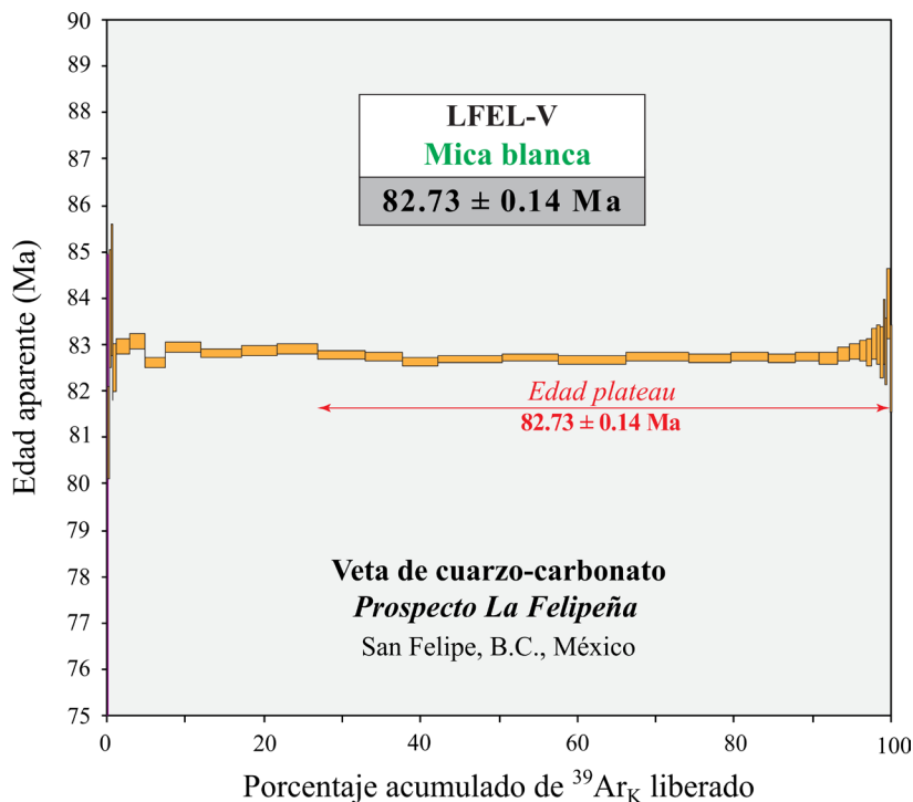
Figura 5 Espectro ^{40}\text{Ar}/^{39}\text{Ar} de calentamiento gradual de hojuelas de mica blanca hidrotermal colectadas en la salbanda de alteración de una veta aurífera de cuarzo-carbonato del prospecto La Felipeña.
