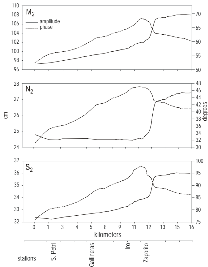
Figure 3. Amplitude, in cm (solid line), and phase, in degrees (dashed line), for the M_2 , N_2 and S_2 tidal constituents along the Sancti Petri Channel. Figura 3. Amplitudes en cm (línea sólida) y fase en grados (línea punteada) para las componentes de marea M_2 , N_2 y S_2 a lo largo del Caño de Sancti Petri.
