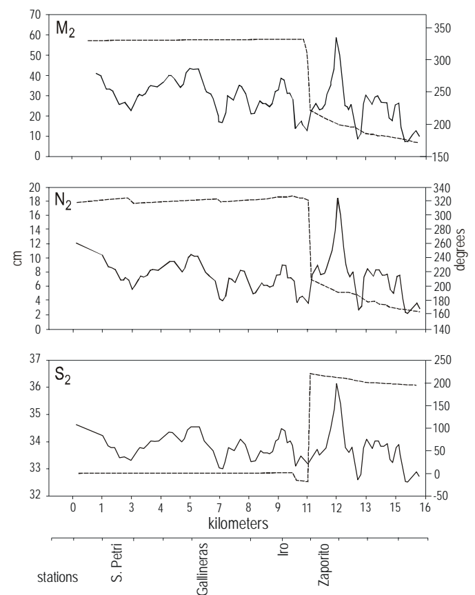
Figure 4. Velocity amplitude, in \text{cm s}^{-1} (solid line), and velocity phase, in degrees (dashed line), for M_2 , N_2 and S_2 along the Sancti Petri Channel. Figura 4. Amplitudes de la velocidad en \text{cm s}^{-1} (línea sólida) y fases en grados (línea punteada) para M_2 , N_2 y S_2 a lo largo del Caño de Sancti Petri.
