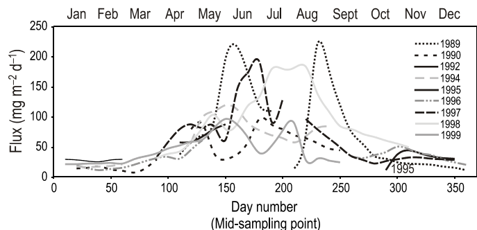
Figura 6. Flujo anual descendente de fitodetrítus en la Planicie Abisal Porcupine de 1989 a 1999 a 3000 m (tomado de Lampitt et al. 2003).
