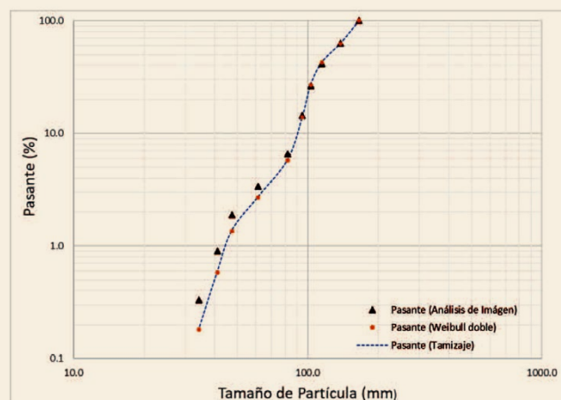
Figura 4. Gráfico de tamaño de partícula versus Pasante (%).
