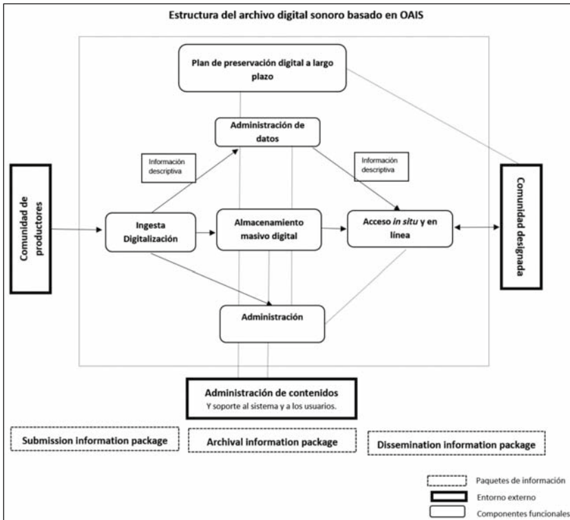
Figura 3. Fuente: elaboración basada en el modelo OAIS
