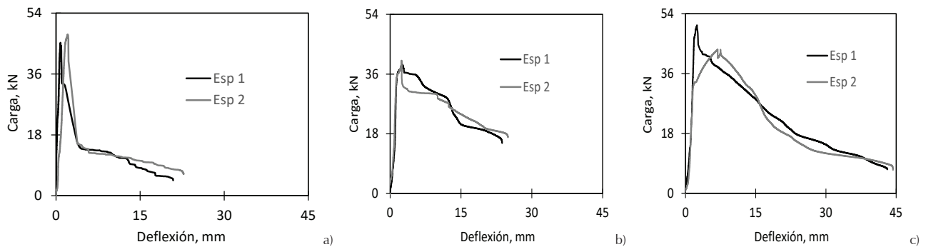
Figura 10. Curvas carga-deflexión de losas de CRFA: a) D_f = 3.4 \text{ kg/m}^3 , b) D_f = 7.6 \text{ kg/m}^3 , c) D_f = 14.1 \text{ kg/m}^3
