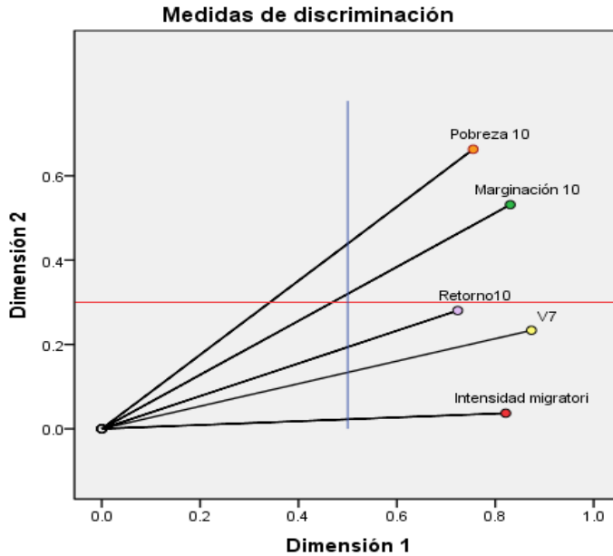
Figura 1: Medida de discriminación de 2010
