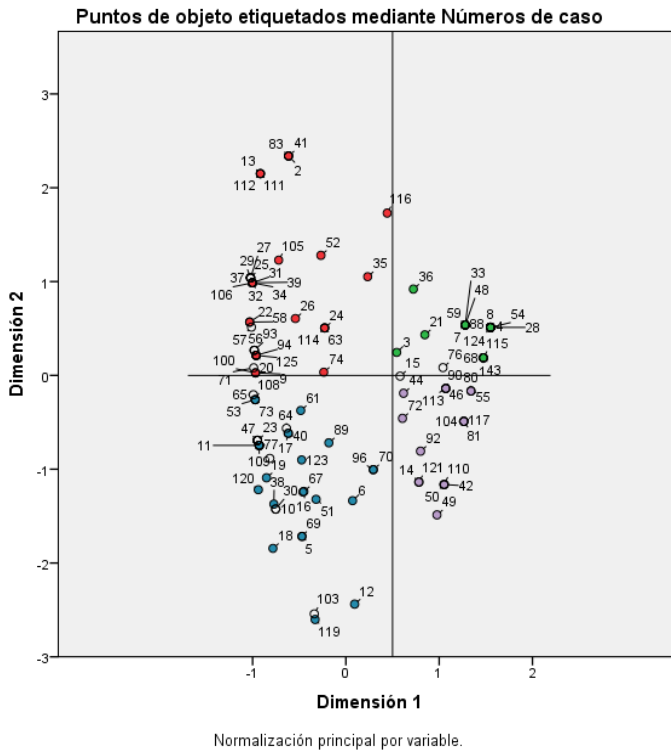
Figura 3: Centroides y objetos del diagrama de dispersión biespacial 2010
