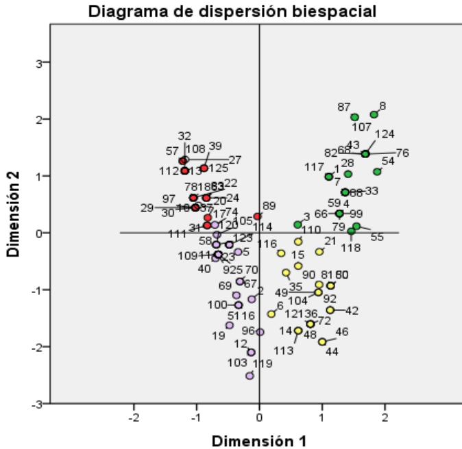
Figura 4: Centroides y objetos del diagrama de dispersión biespacial 2015
