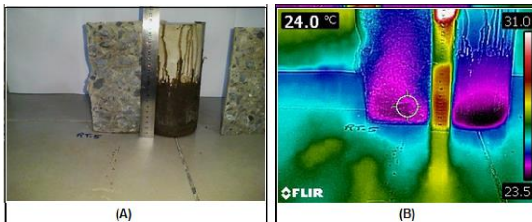
Figura 10. Imagen termográfica infrarroja para la serie con resina termoplástica. A - Probeta luego del ensayo de compresión diametral; B - Probeta durante el ensayo de termografía .
